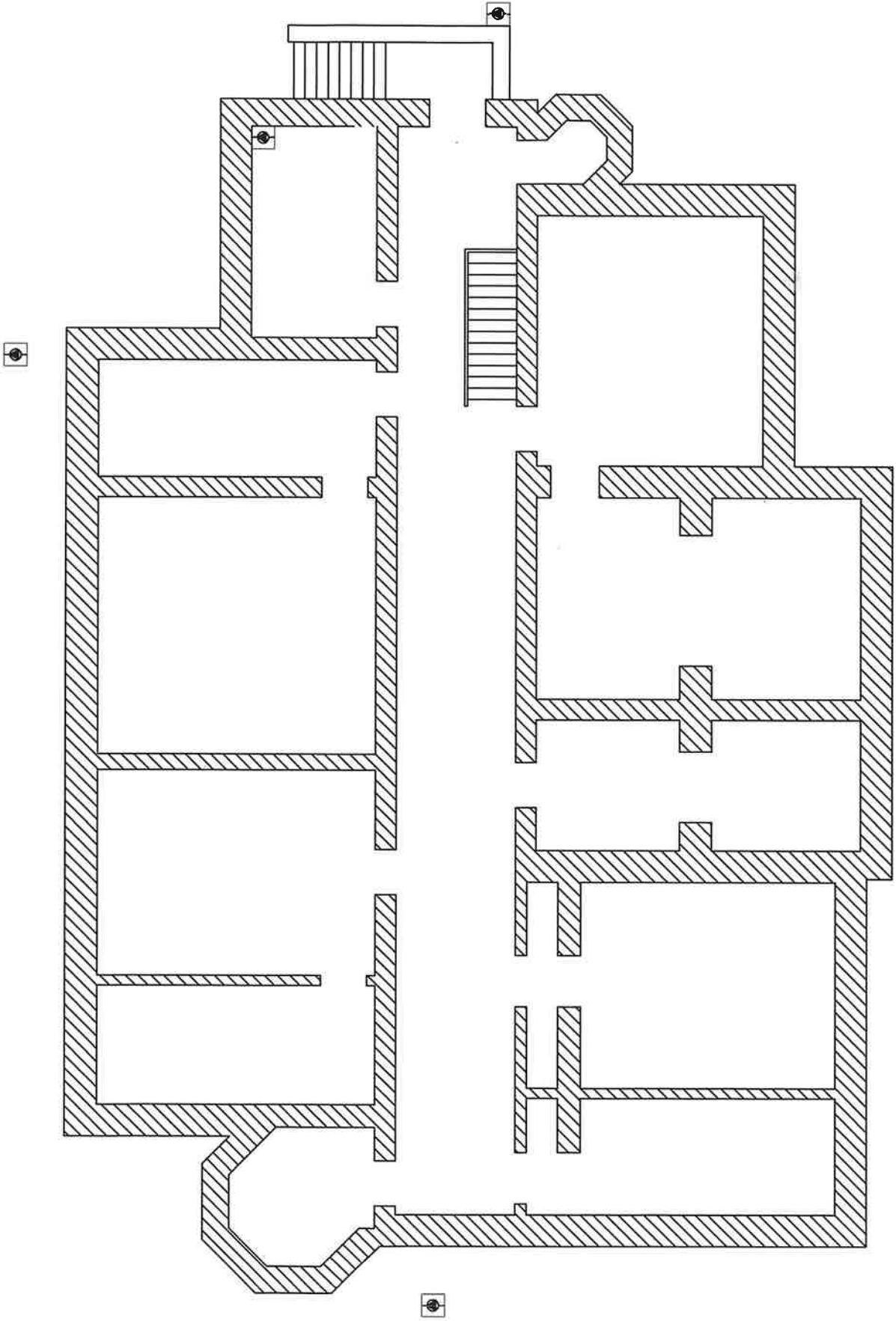
grondplan kelder Blauwendaal schaal 1/100
